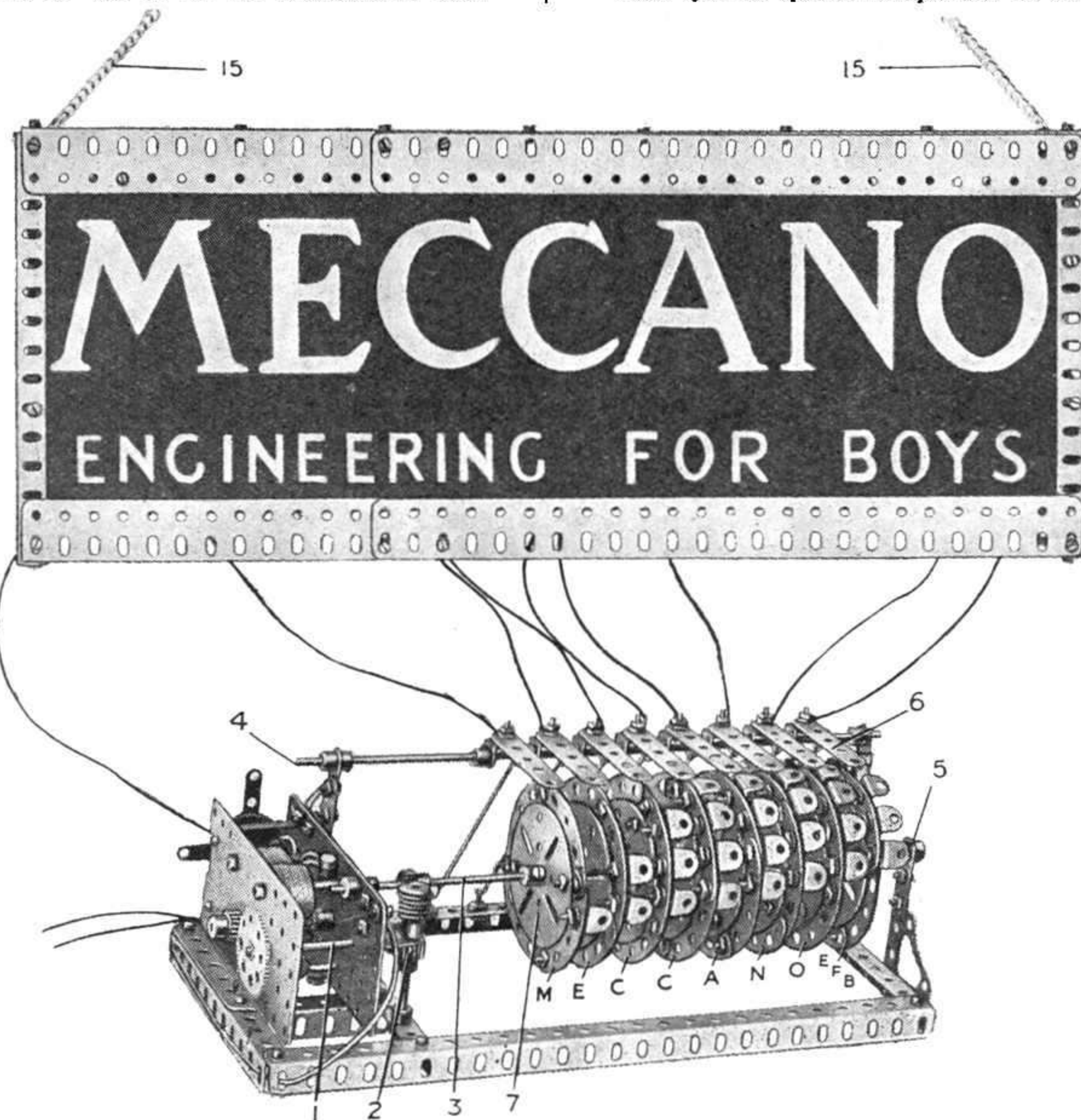
Fig. 1. — Vue générale de l'Enseigne Lumineuse Meccano
