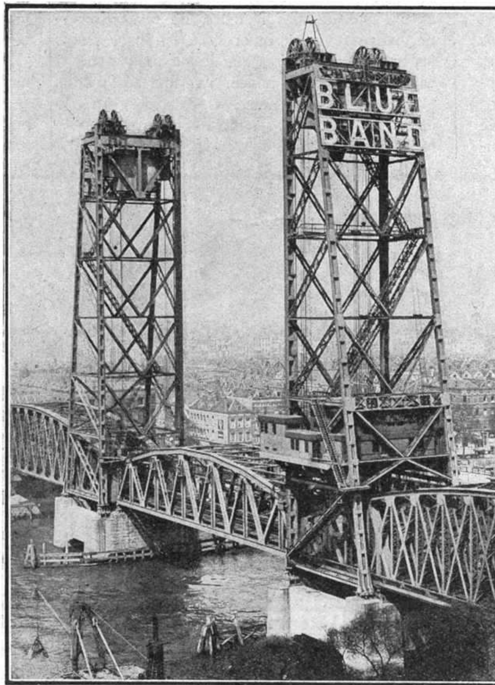
Le Pont-Levant de Rotterdam, vue du Pont, la Travée du milieu abaissée
