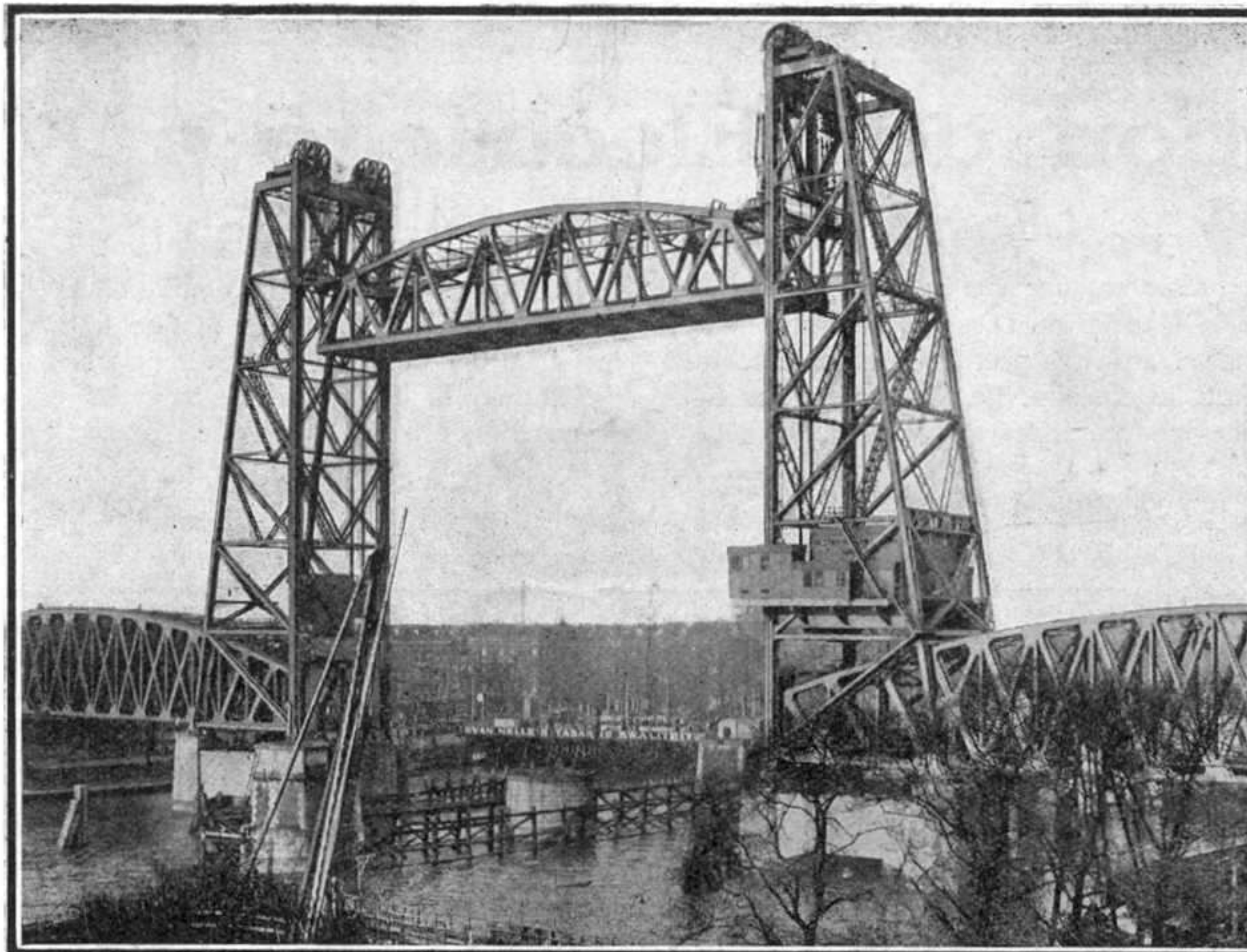
Le Pont Levant de Rotterdam. Vue du Pont, la Travée relevée. On voit, entre les deux pylones, la pile Centrale de l'ancien Pont-Tournant
