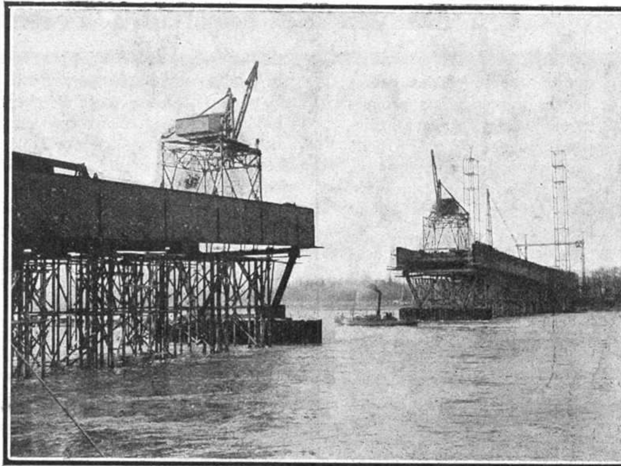
Un Pont Géant sur le Rhin Ce Pont, dont les travaux sont très activement poussés, réunira les deux rives du Rhin près de Mulheim. La longueur sera de 550 mètres
