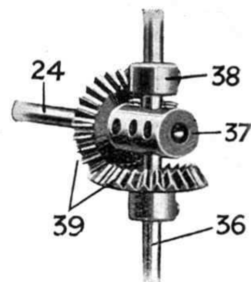
Fig. 4. — Mécanisme commandant les Voitures tournantes
