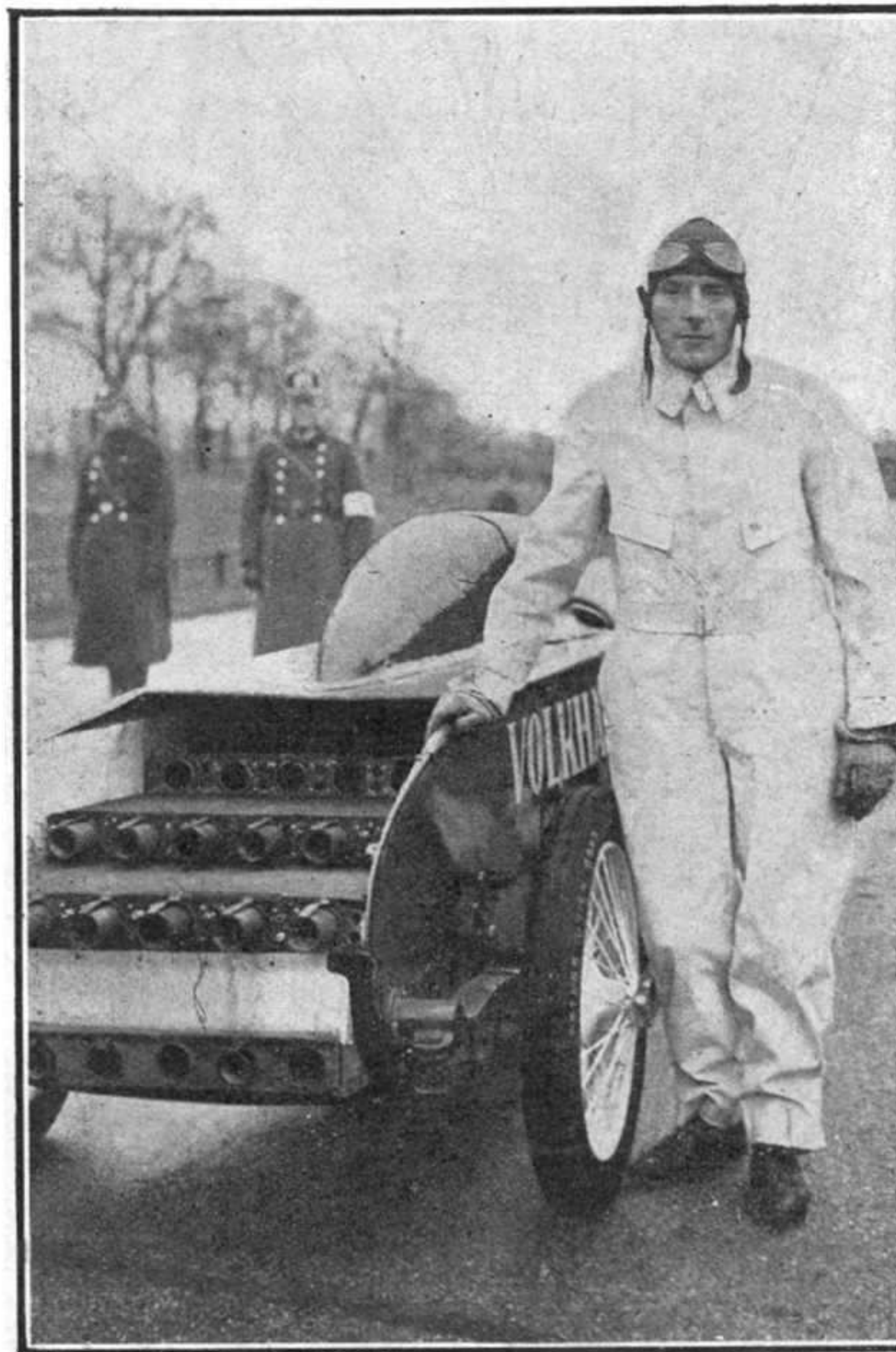
Une nouvelle Autofusée. Cette nouvelle auto, de Volkhart, vient d'être expérimentée à Berlin
