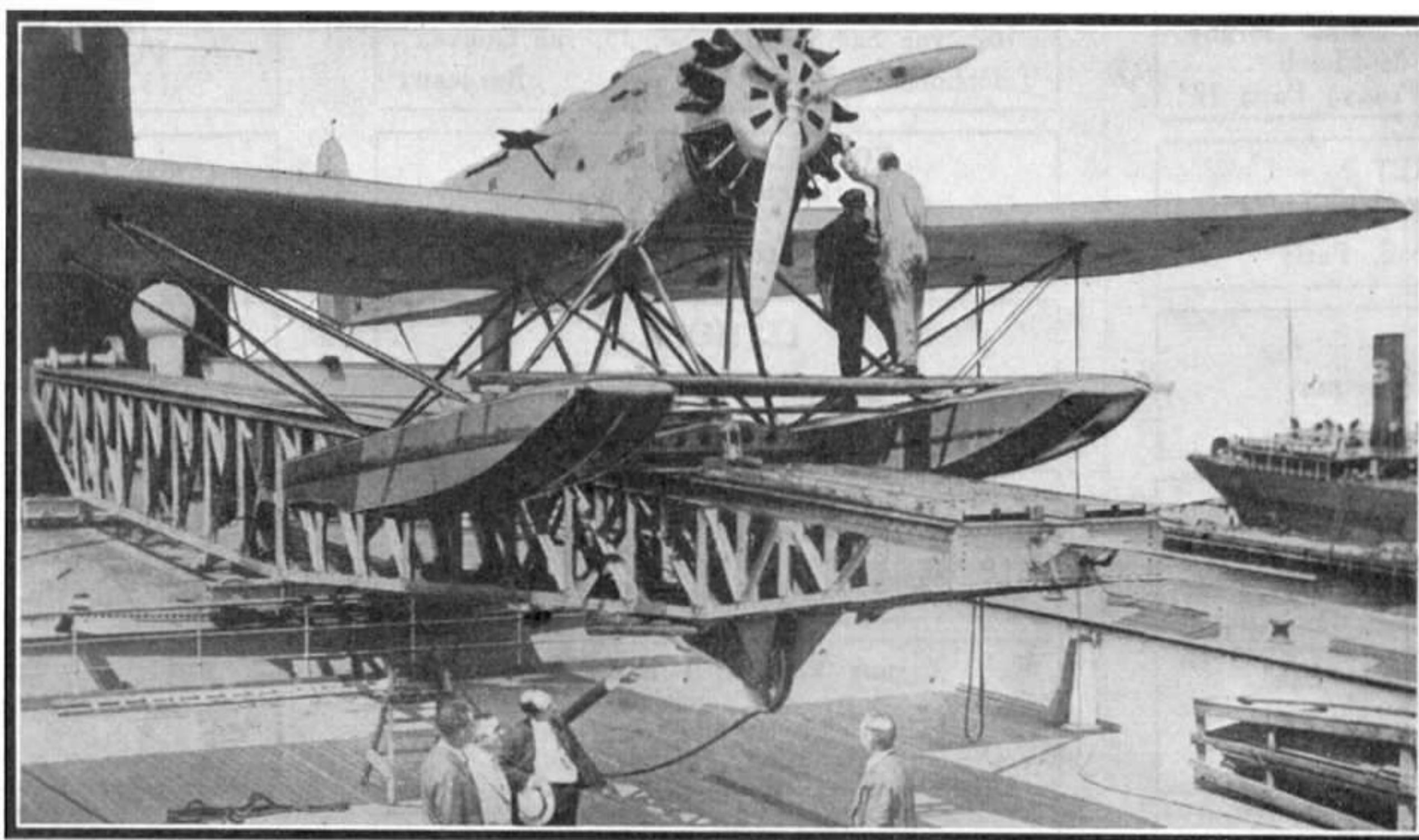
Hydravion en position de lancement sur la catapulte installée à bord du transatlantique « Bremen »
