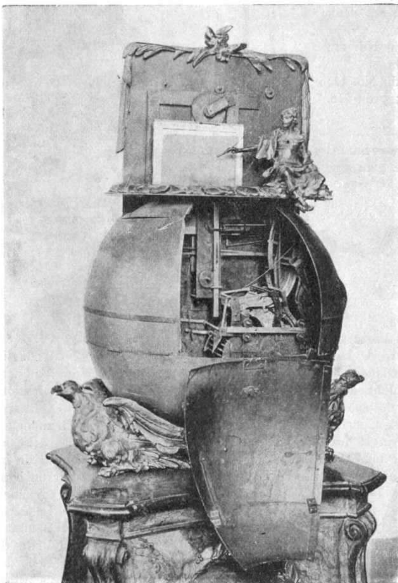
Automate écrivant construit en 1760 par Fr. Knauss
