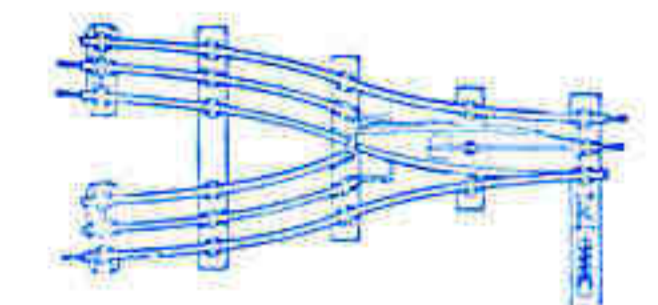
EPFR2 Aiguillages Parallèles Electriques (de droite)
