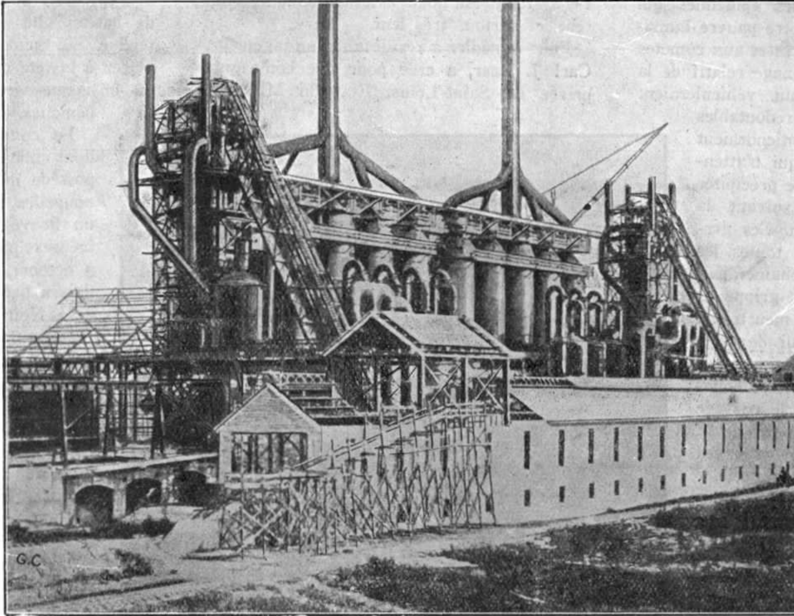
Ensemble de deux hauts fourneaux modernes.
