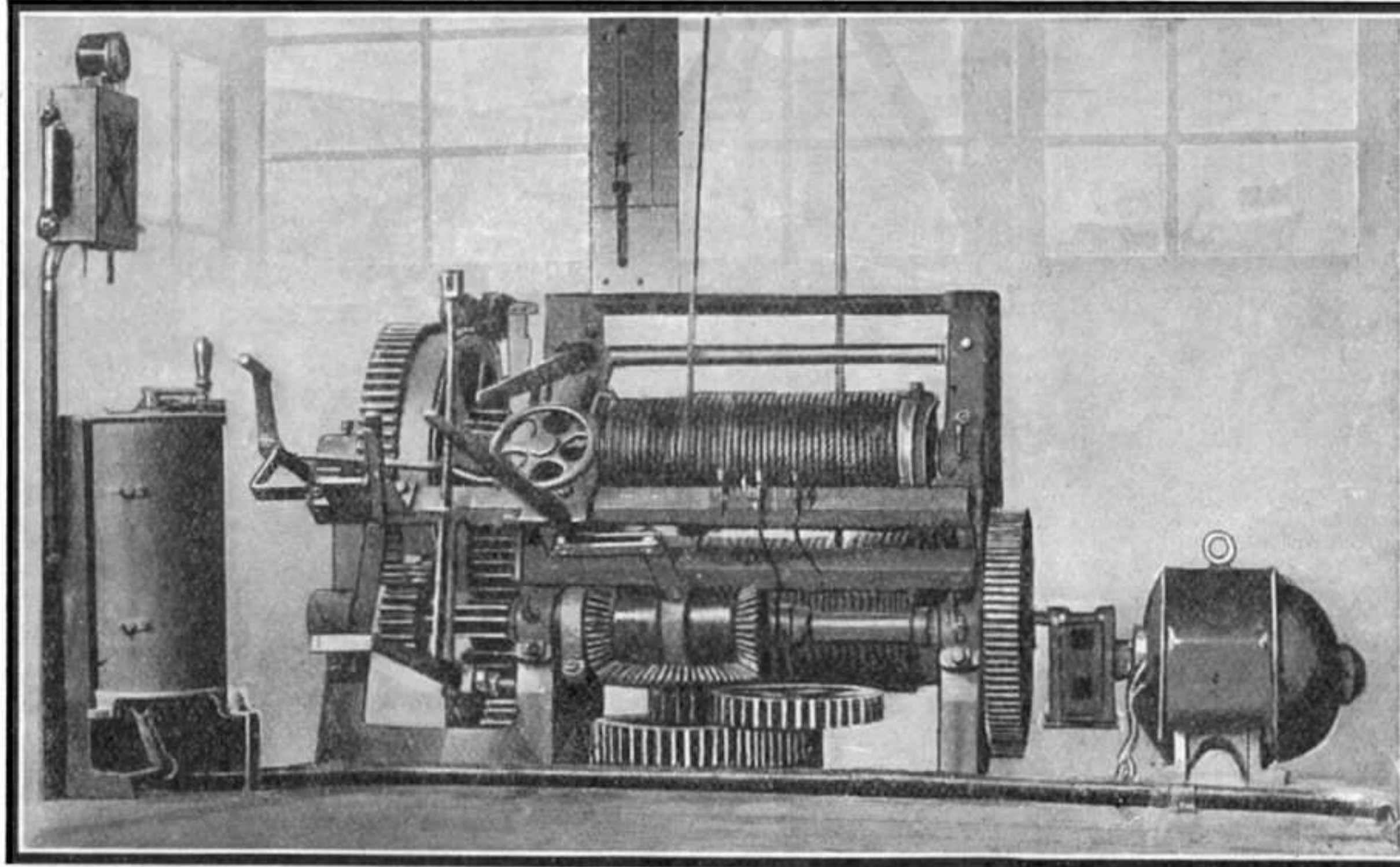
Fig. 3. — La machinerie d'une véritable grue Derrick électrique.
