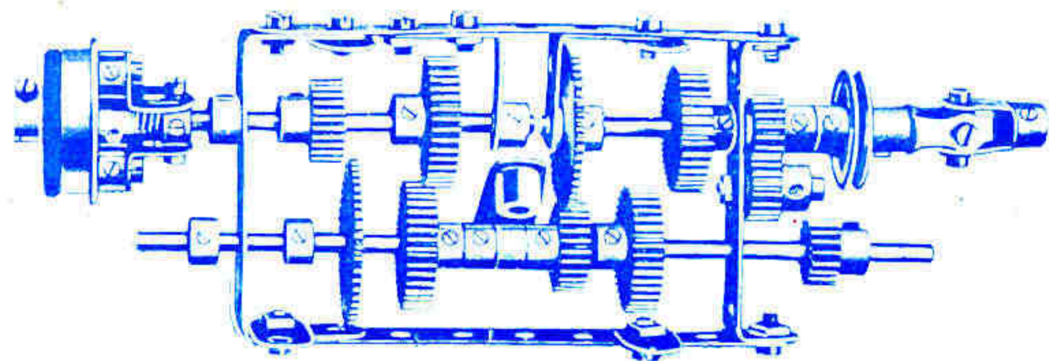
BOITE DE VITESSE "MECCANO" ET EMBRAYAGE
