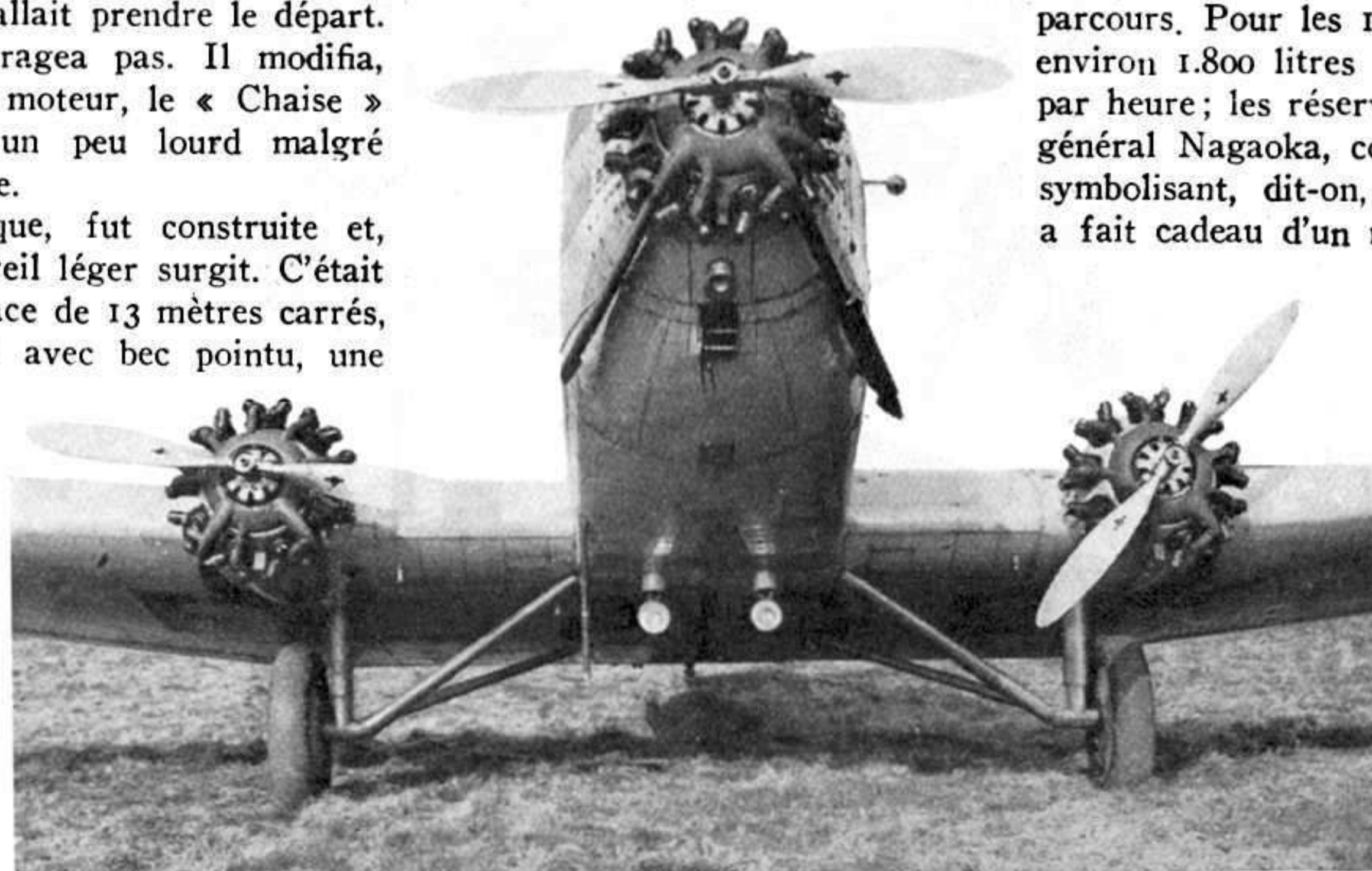
Le Wibault-Penhoët 281-T.12 muni de 3 moteurs Gnome-Rhône K7B et aménagé pour 10 passagers, est l'avion trimoteur de transport le plus rapide du monde.
