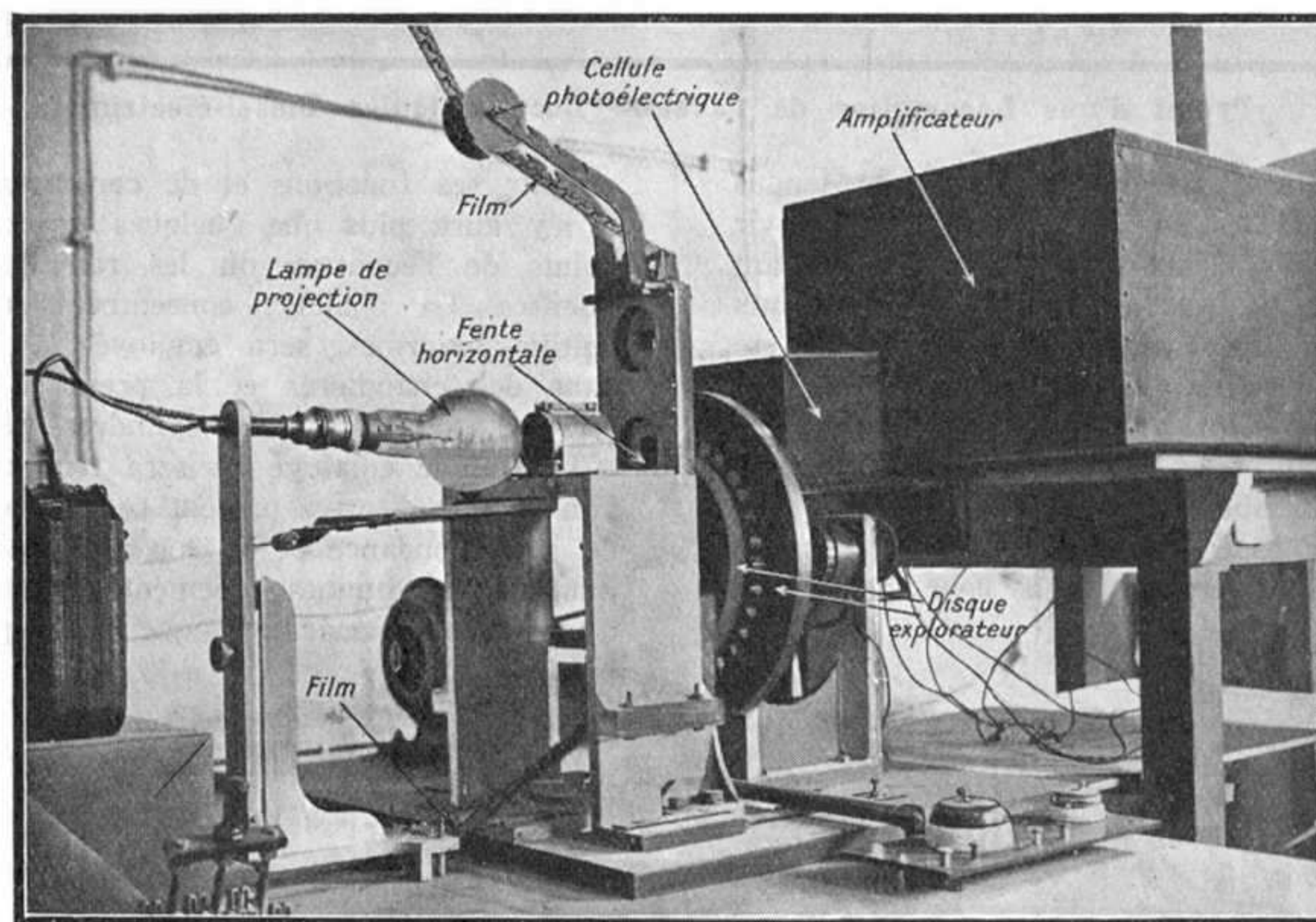
Le Télécinéma Barthélémy: Poste de Transmission.
