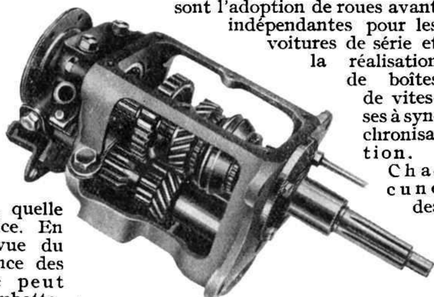
Vue intérieure de la nouvelle boîte de vitesses Citroën, montrant les engrenages silencieux et le mécanisme synchroniseur. Cette photo, ainsi que celle du mécanisme de roue libre (page ci-contre), nous a été confiée par les Etablissements Citroën.
