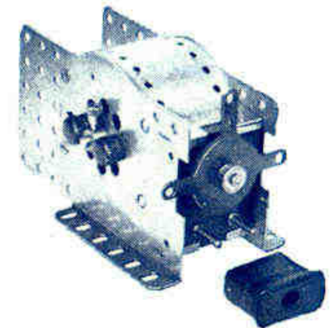
Moteur Electrique N° 2 110 et 220 volts
