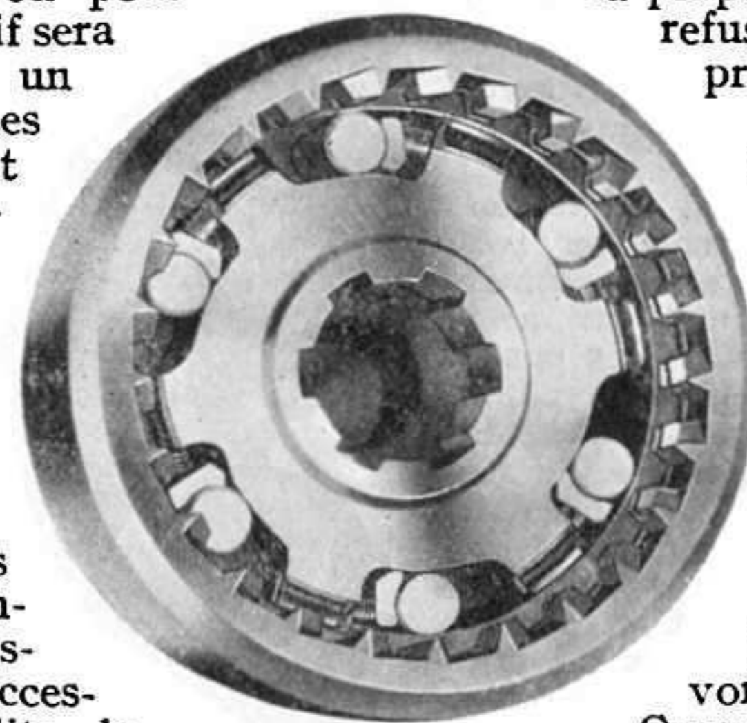
Vue intérieure du mécanisme de la roue libre Citroën.
