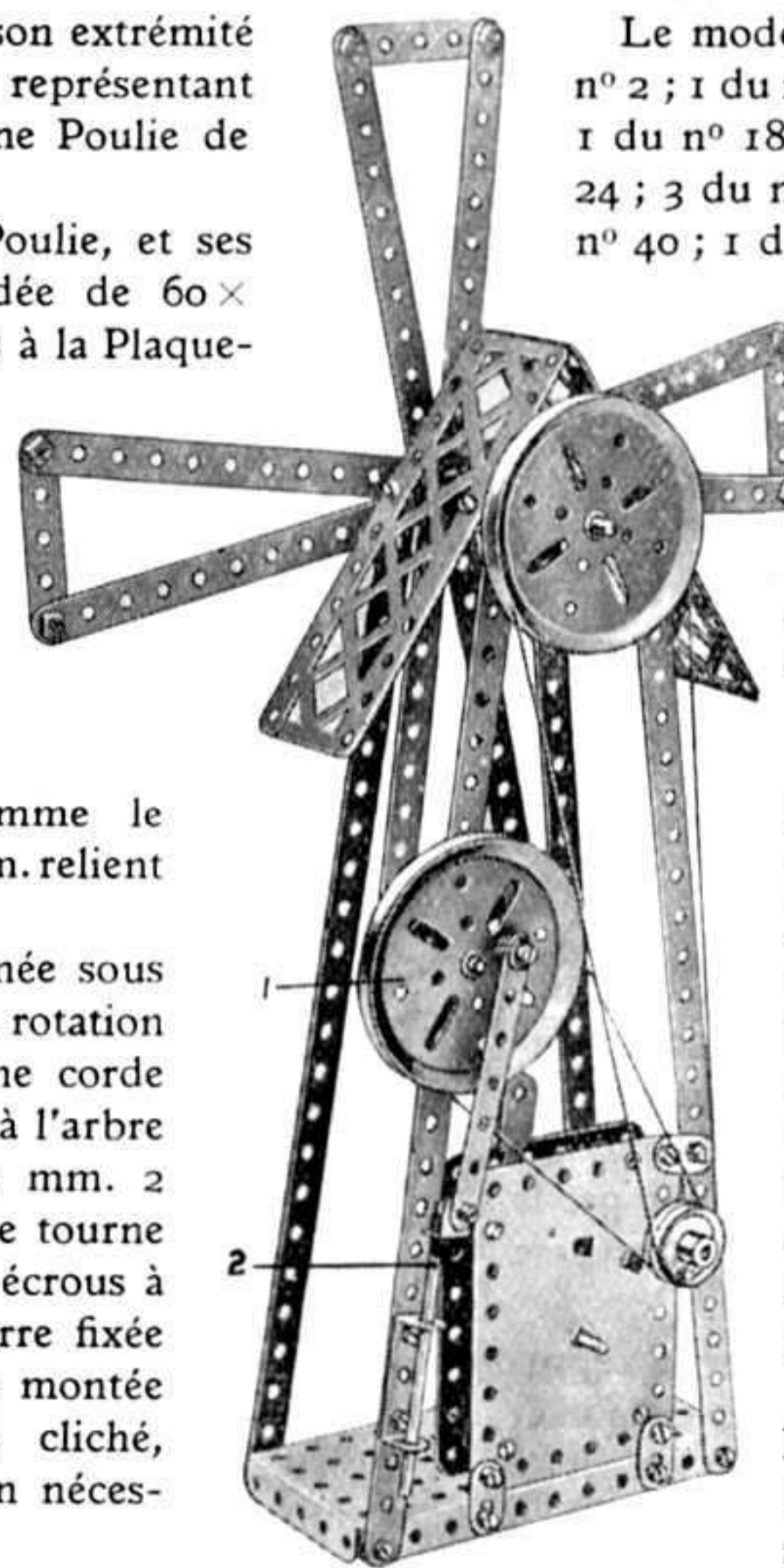
Fig. 4. Pompe éolienne
