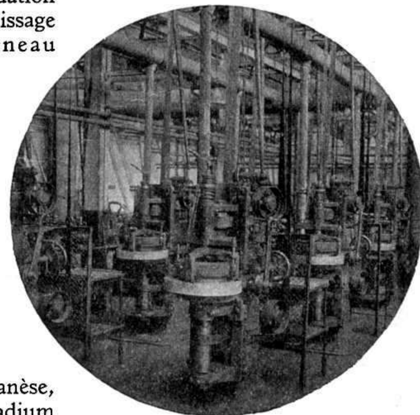
Atelier de dégrossissage des billes avant trempe.
