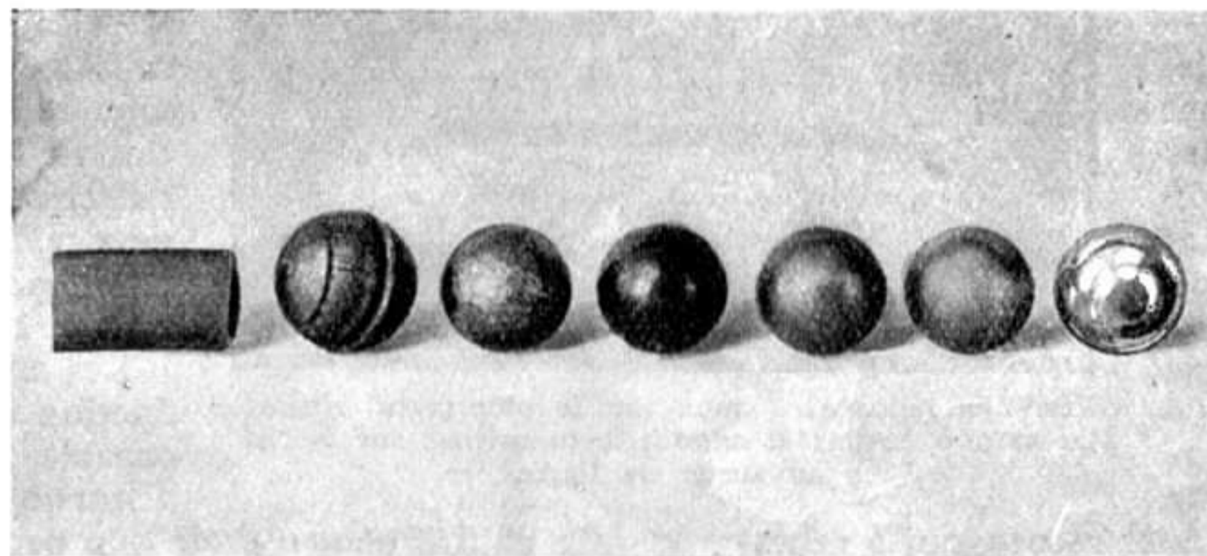
Les phases successives de fabrication d'une bille.
