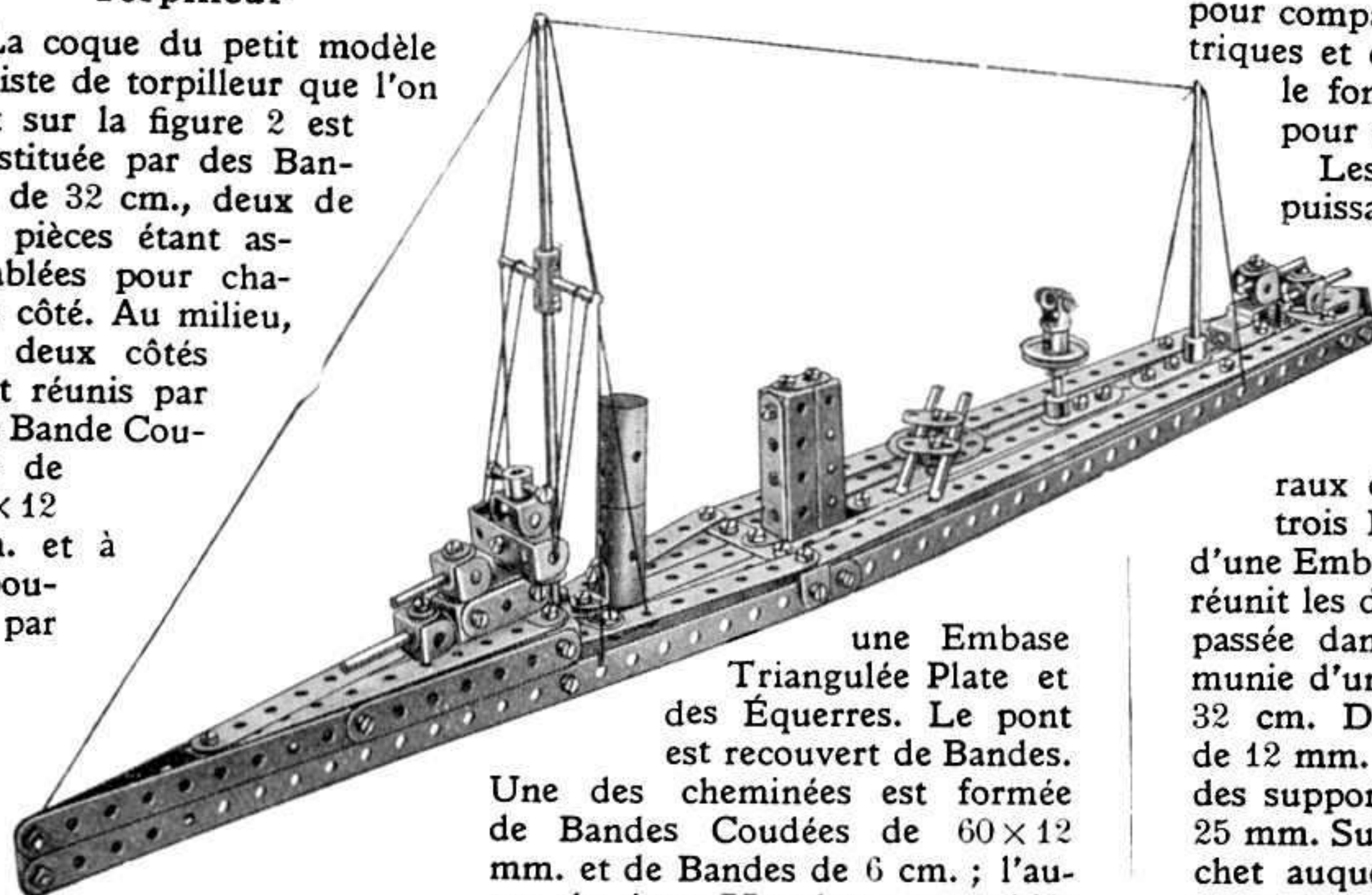
Fig. 2. — Torpilleur.
