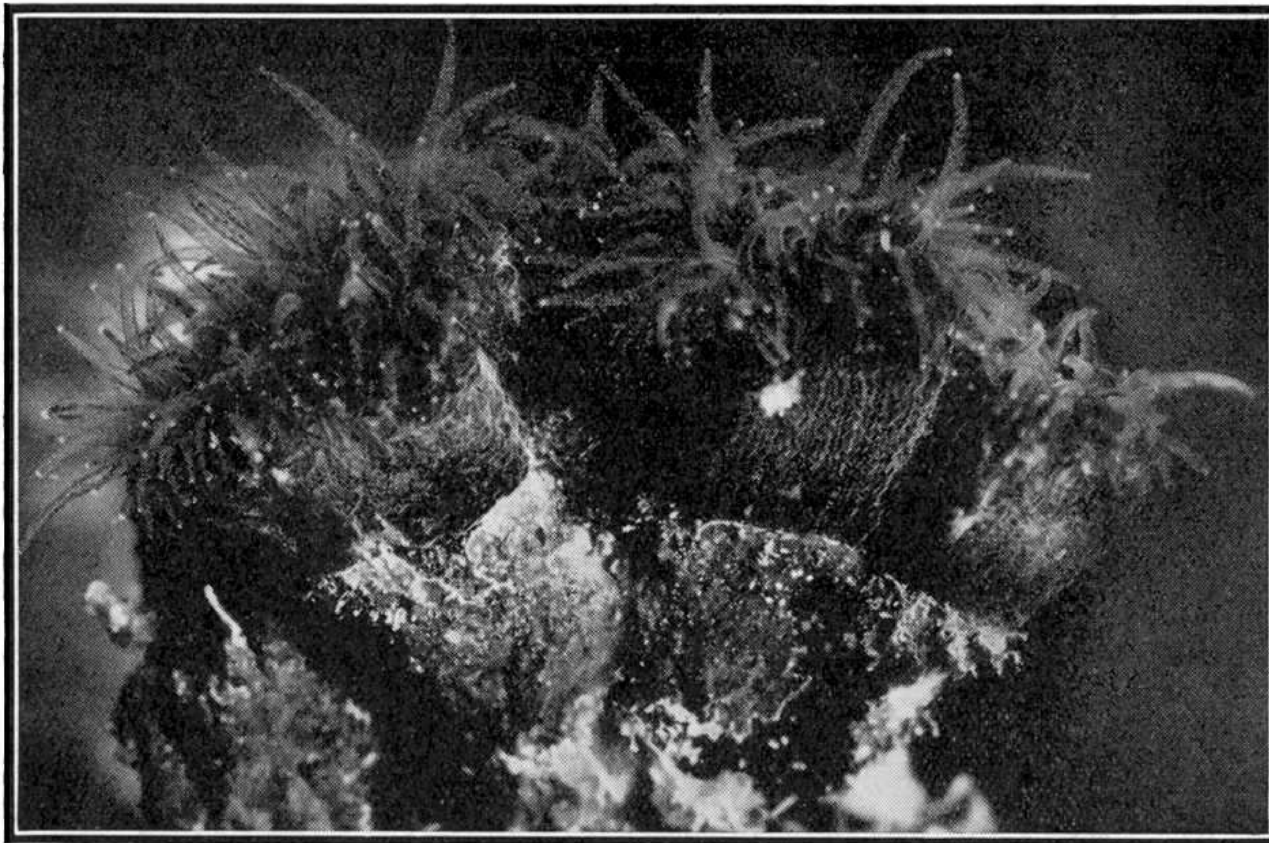
Polypier de corail photographié à Tortuga. On remarque, en haut, la frange de tentacules des madreporae vivants.
