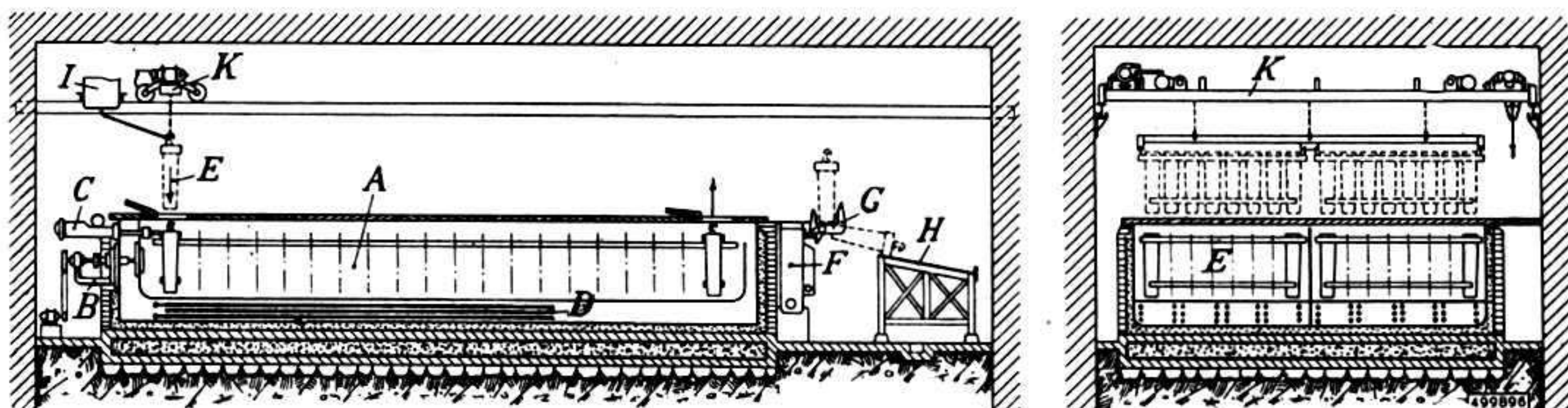
Coupes longitudinale et transversale d'un générateur à glace. A. Bac à glace. — B. Agitateur à hélice. — C. Avancement automatique. — D. Serpents évaporateurs. — E. Rame de mouleaux. — F. Bac de démoulage. — G. Basculeur. — H. Table de démoulage. — I. Remplisseur automatique. — Q. Pont roulant.
