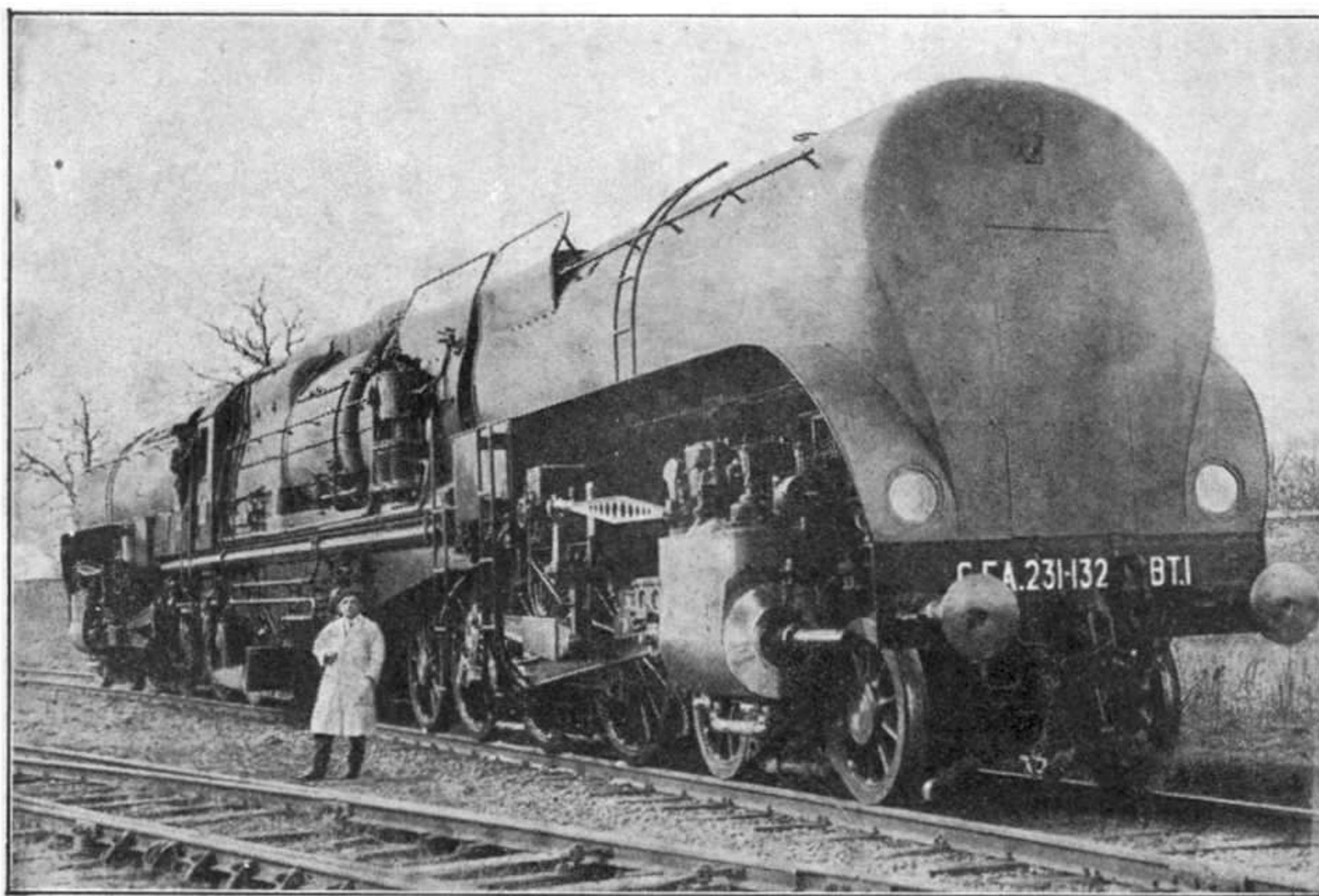
La locomotive Garratt des Chemins de fer algériens, au cours des essais. En haut de la page — elevation de la locomotive. (A, réservoir d'eau ; B, arbre de changement de marche ; C, prises d'air auxiliaires ; D, turbo-générateurs d'éclairage et de changement de marche ; E, pousseur de charbon à vapeur ; F, chaudière.)
