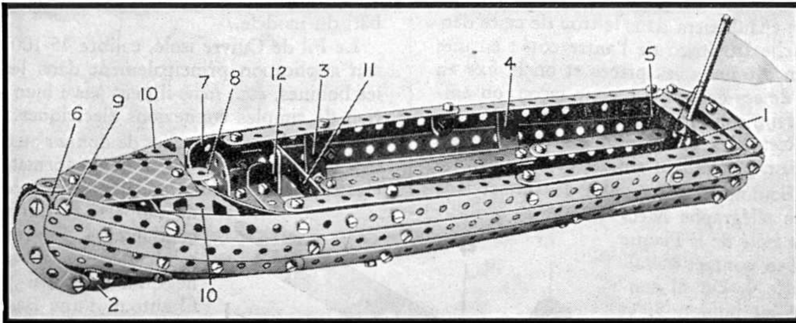
Fig. 1. — Chaloupe à moteur.
