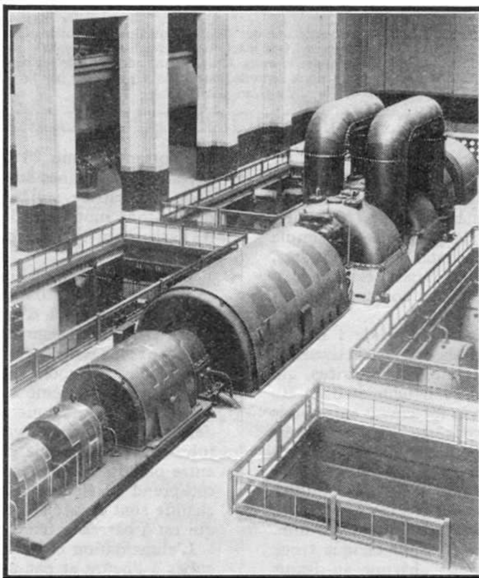
Vue générale du groupe turbo-alternateur de 105.000 kW.
