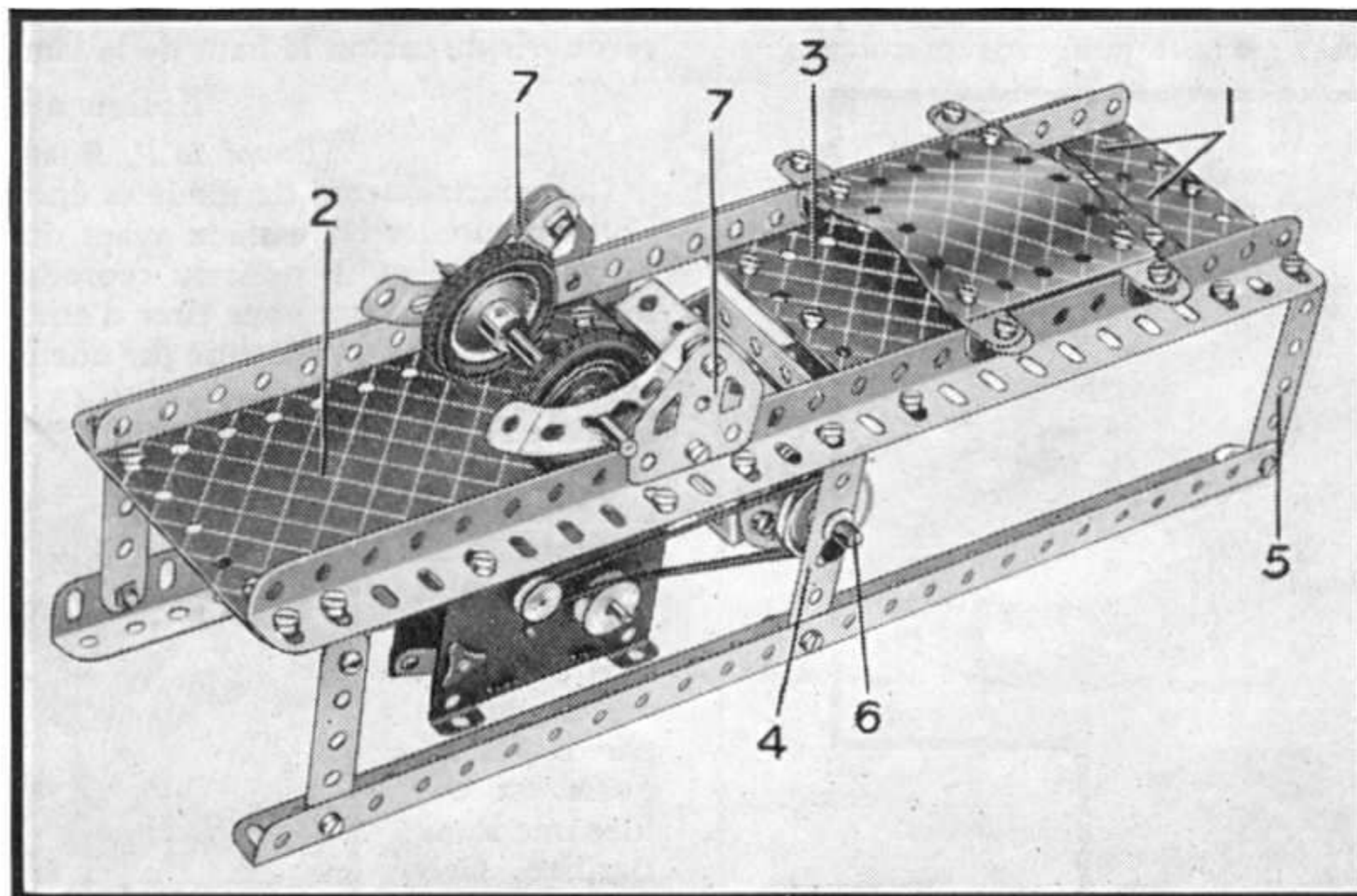
Fig. 1. — Raboteuse.
