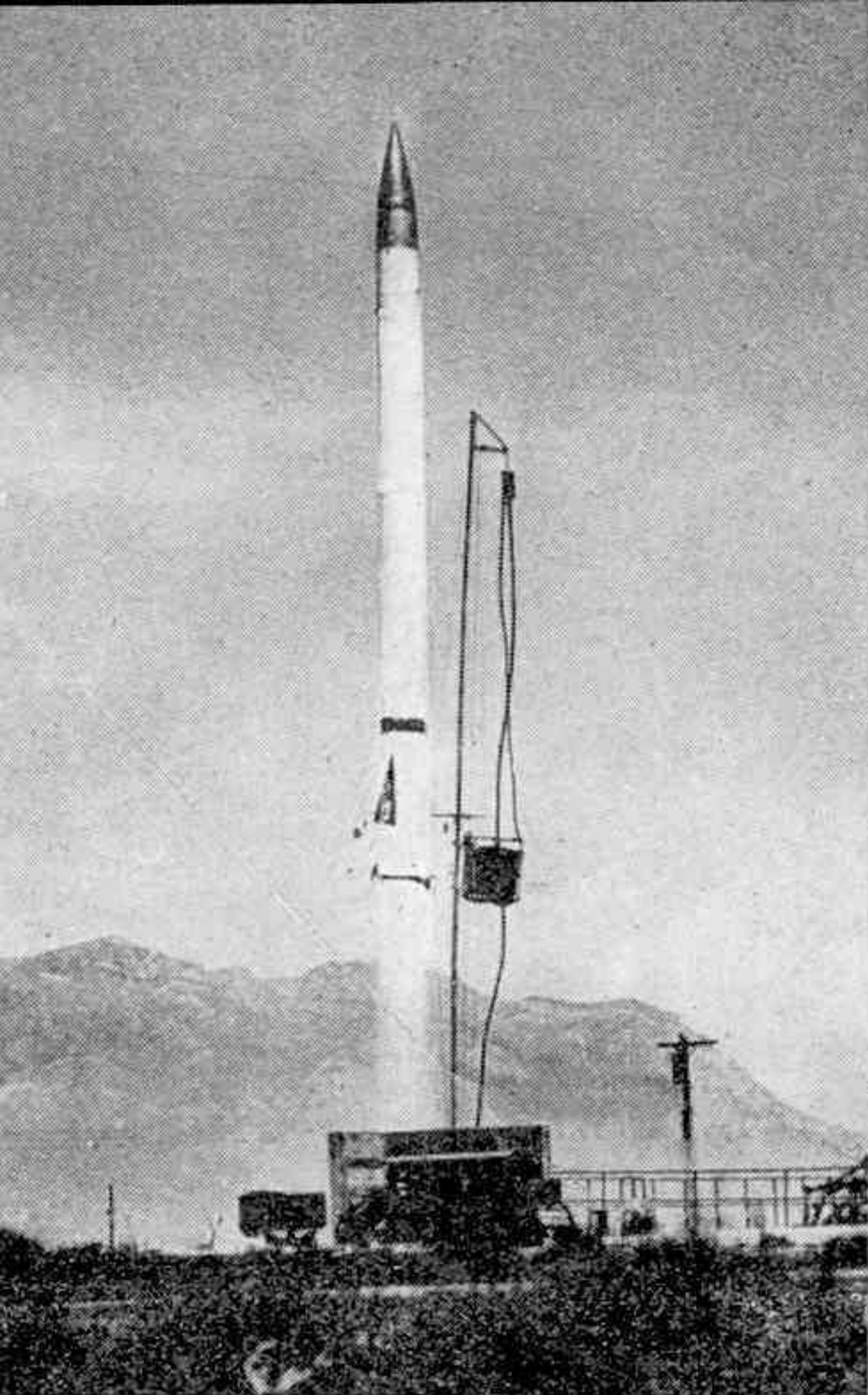
Le « Viking », fusée américaine propulsée par alcool éthylique et oxygène liquide, a atteint l'altitude de 216 kilomètres. Elle pèse 4 t ,5 et mesure 14 mètres de longueur sur 0 m ,81 de diamètre.
