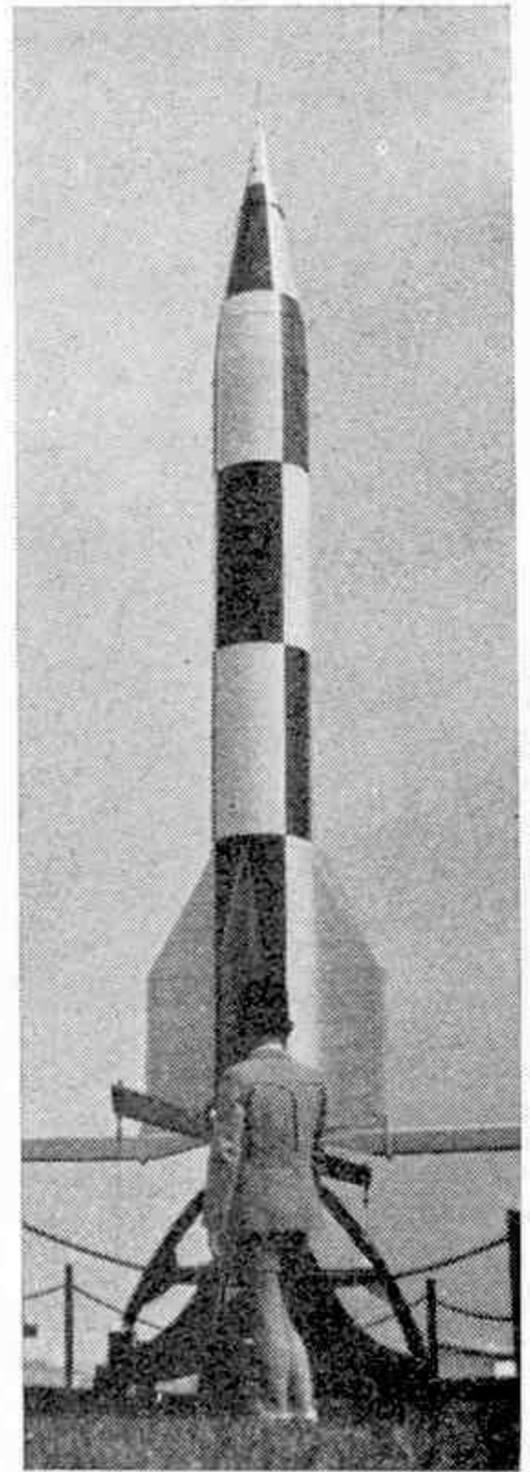
« Véronique », fusée française construite par le laboratoire de balistique et d'aérodynamique de Vernon, est chargée de l'exploration de l'atmosphère supérieure (jusqu'à 125 kilomètres).
