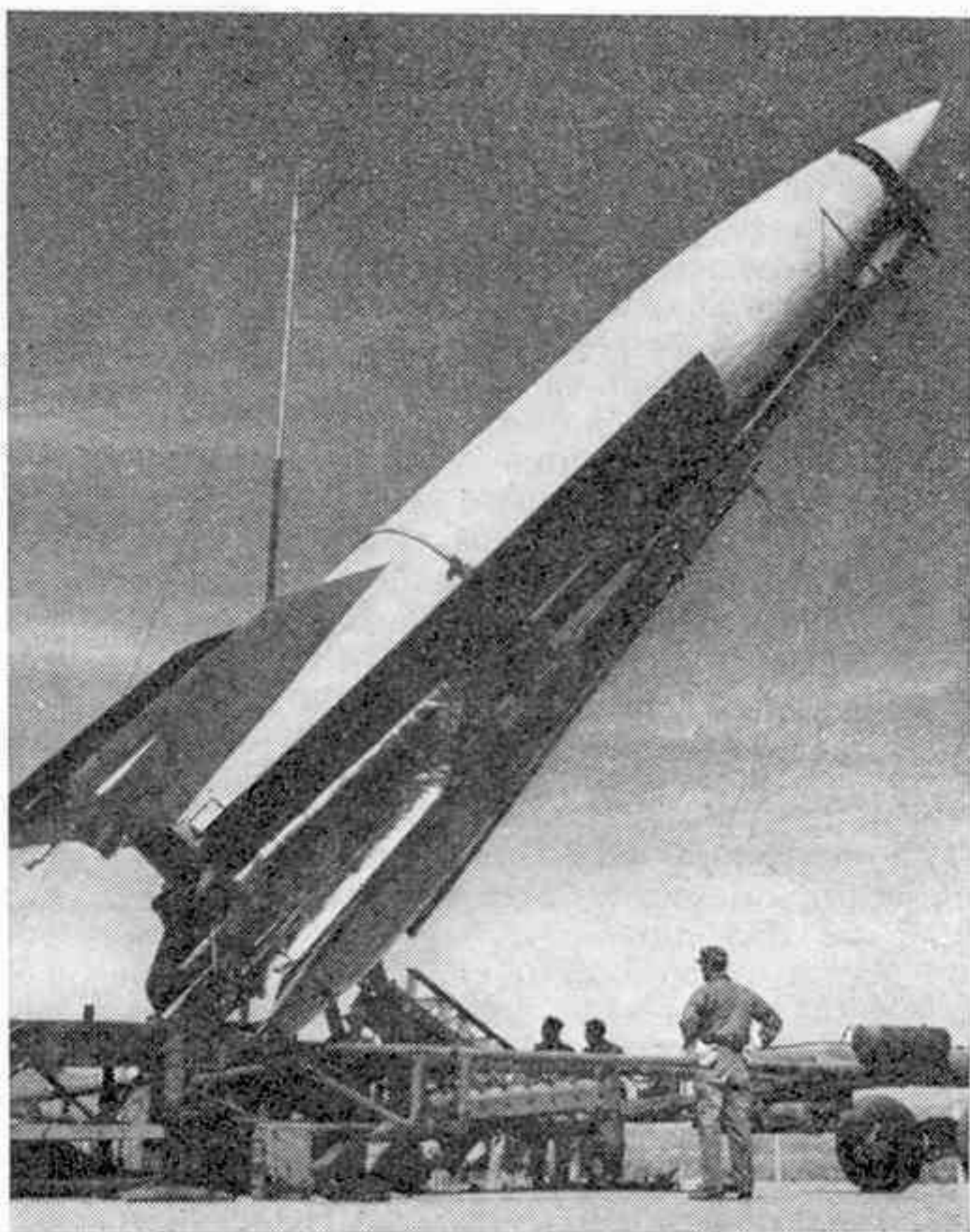
Mise en place d'une fusée américaine V2 sur sa rampe de lancement. C'est un engin de ce type qui portait, en gigogne, la fusée Wac Corporal qui battit, avec 402 kilomètres, le record d'altitude.
