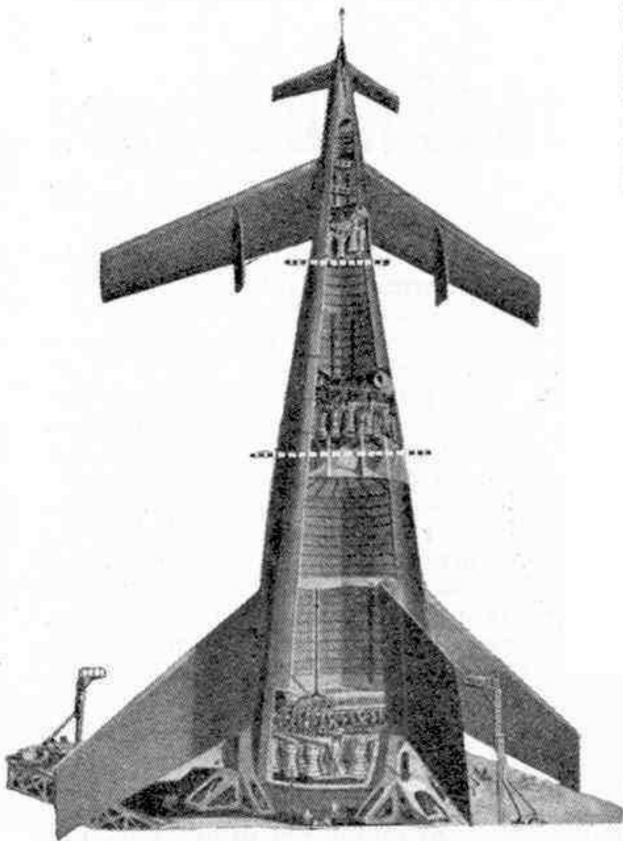
RÉALITÉ DE DEMAIN : Projet de fusée glogone à trois étages du Dr Von Braun. Seul l'élément supérieur porte l'équipage et parviendra à vaincre la force d'attraction terrestre. Les pointillés séparent les trois éléments. (D'après Colliers.)
