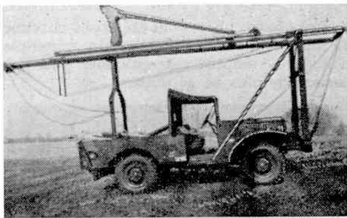
Les deux éléments de la grue et la flèche se replient sur le camion pour le transport. Tout le fonctionnement de l'appareil (y compris sa mise en ordre de marche) est commandé par le treuil du camion.
