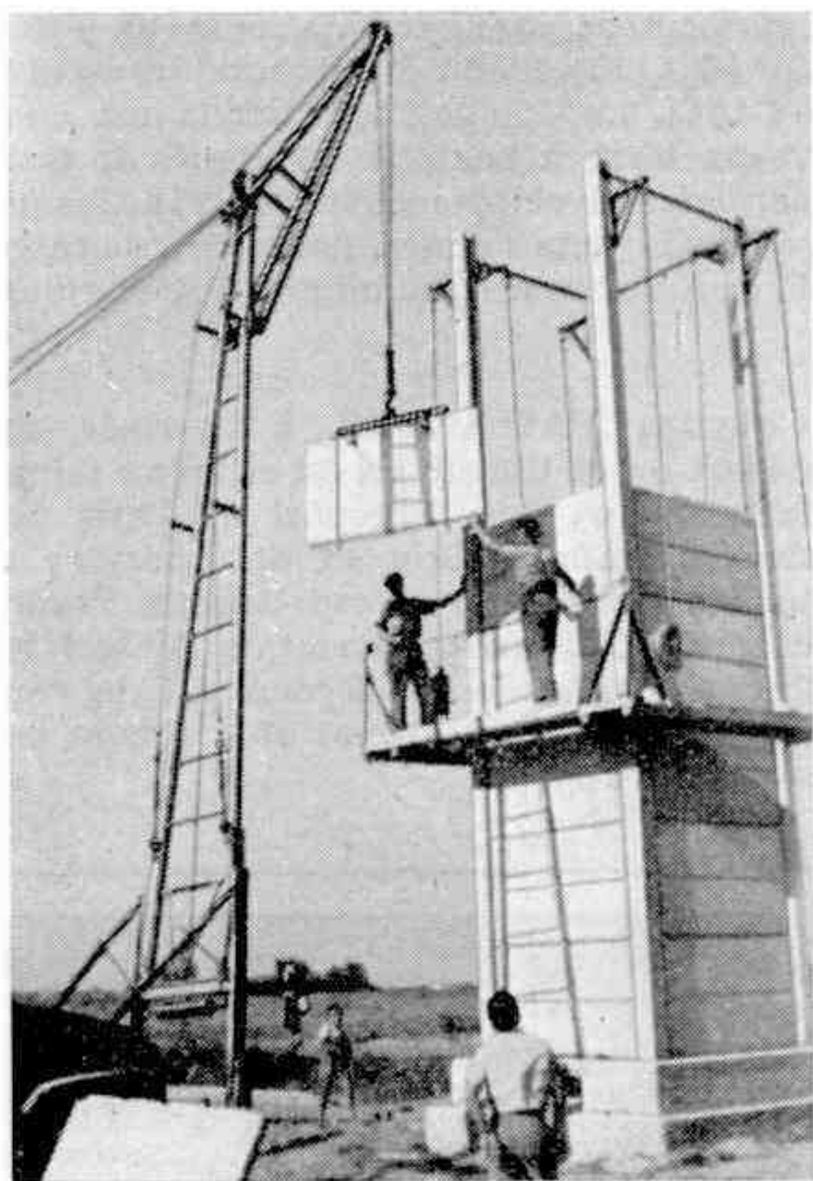
La grue en tube d'acier permet la construction rapide de transformateurs ou la pose de poteaux de ciment. Une plaque de béton comme celle-ci ne pèse que 260 kilogrammes, mais un poteau en pèse 800.
