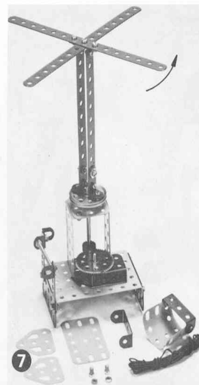
Flying Chairs Carrousel zweefmolen Kettenflieger Karusell Sillas voladoras Giostra a sedici volanti
