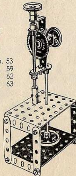
Drilling Machine Machine à Percer
