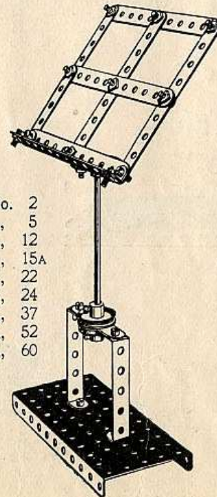
Music Stand Pupitre à Musique
