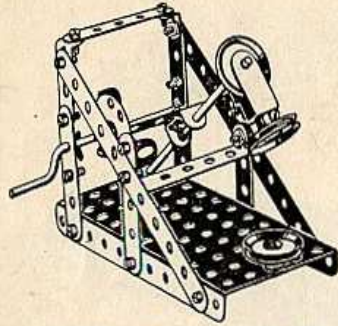
Drop Hammer Marteau à Déclic
