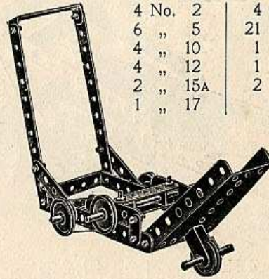
Music Stand Pupitre à Musique
