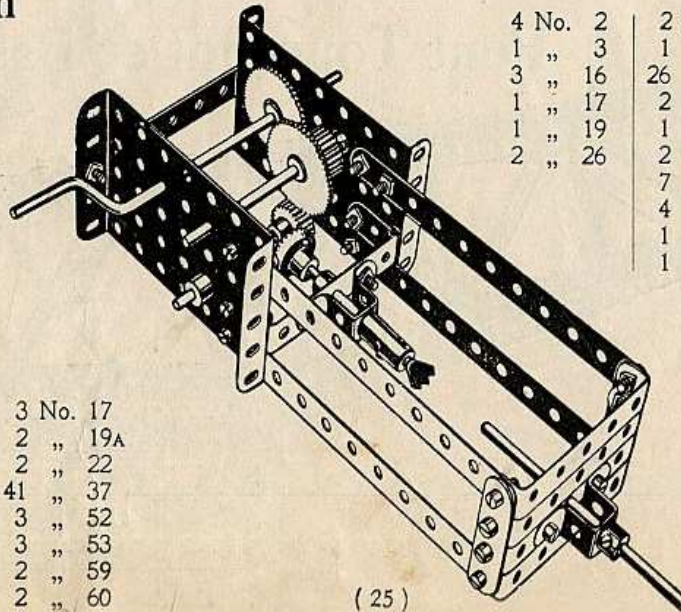
Spooling Machine Bobinoir
