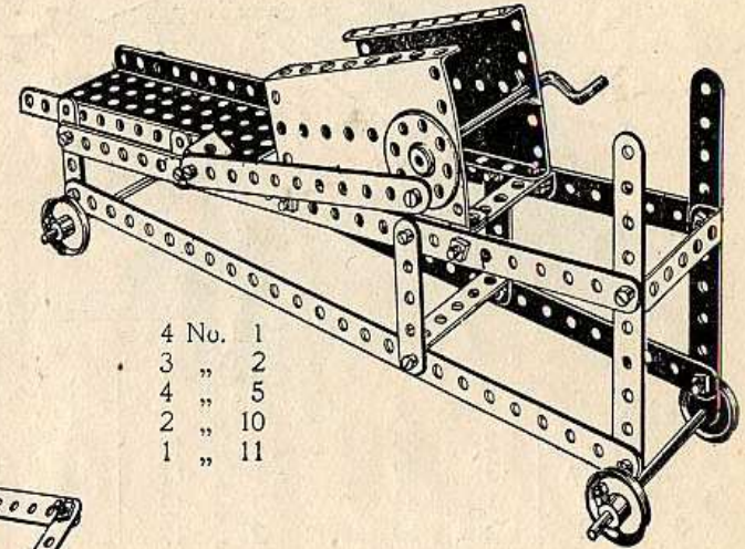
Maize Sheller Décortiqueuse
