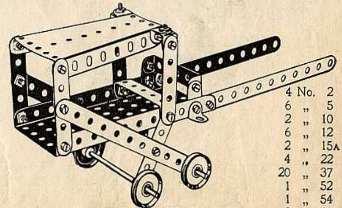
Ticca Gharry Pousse-Pousse Indien
