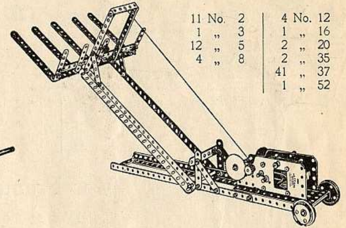
Hay Stacker Faneuse
