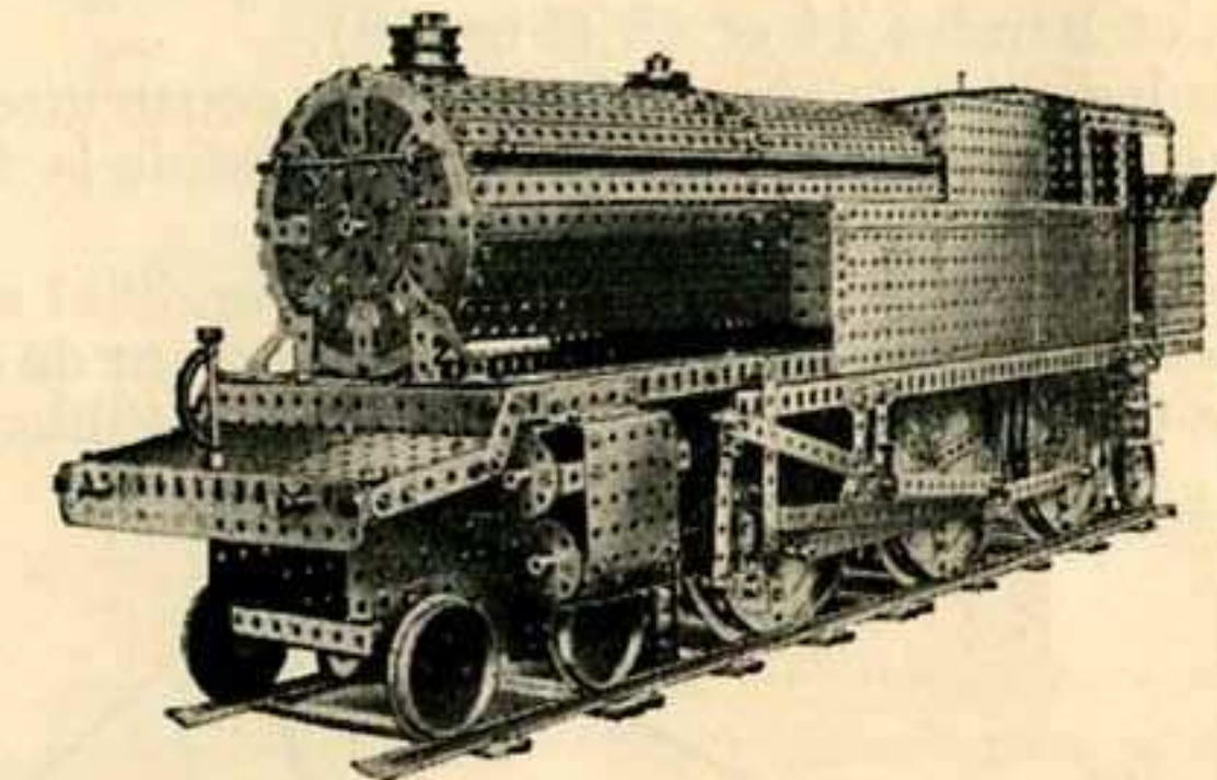
Locomotive Réservoir. Les roues motrices sont actionnées par un Moteur Electrique. Le modèle est muni d'une reproduction exacte du système de soupape Walschaerts. Prix de la feuille spéciale d'instructions Frs. 1.50.
