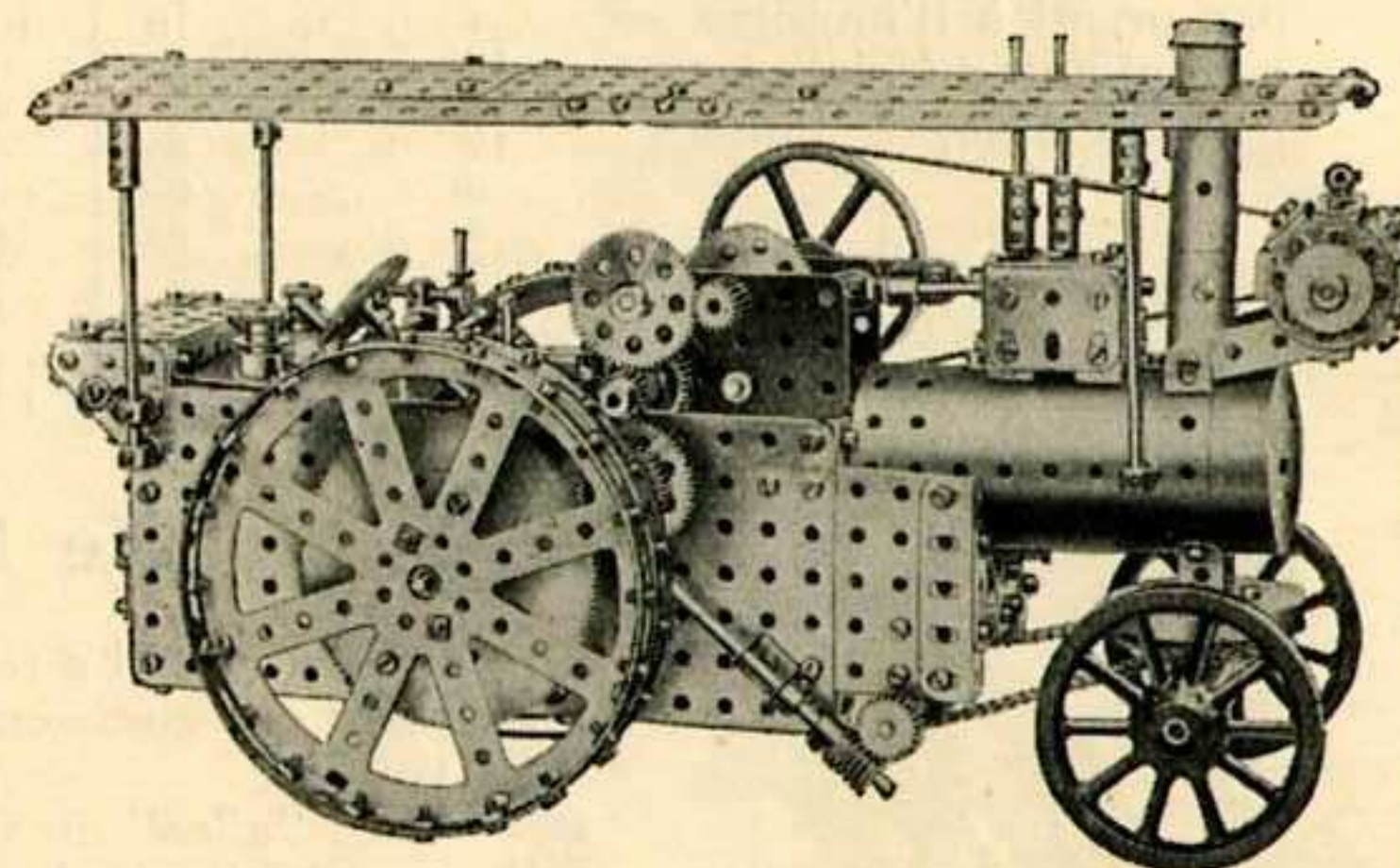
Tracteur à Vapeur. C'est un puissant modèle qui peut remorquer de lourdes charges. Il est actionné par un Moteur de 4 volts et est muni d'une boîte de vitesse, donnant deux vitesses et une marche renversée, d'un arbre de manivelle, d'un piston à soupape, d'une direction à vis sans fin et chaîne, d'un frein, d'une dynamo etc. C'est un bel exemple des dernières créations Meccano. Prix de la Feuille spéciale d'instructions Frs. 1.00.
