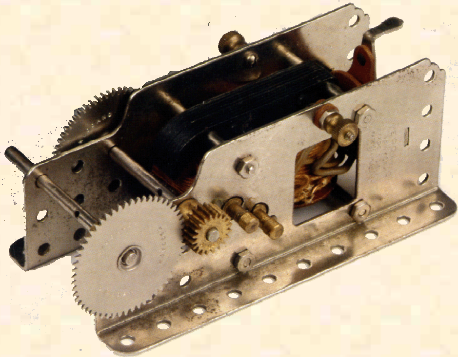
Moteur électrique E2, 4 Volts de 1916 avec sa boîte vente en Amérique
