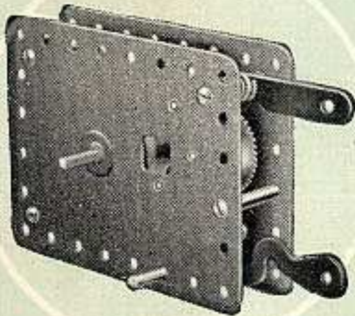
Moteur mécanique No. 1 Veer-motor No. 1
