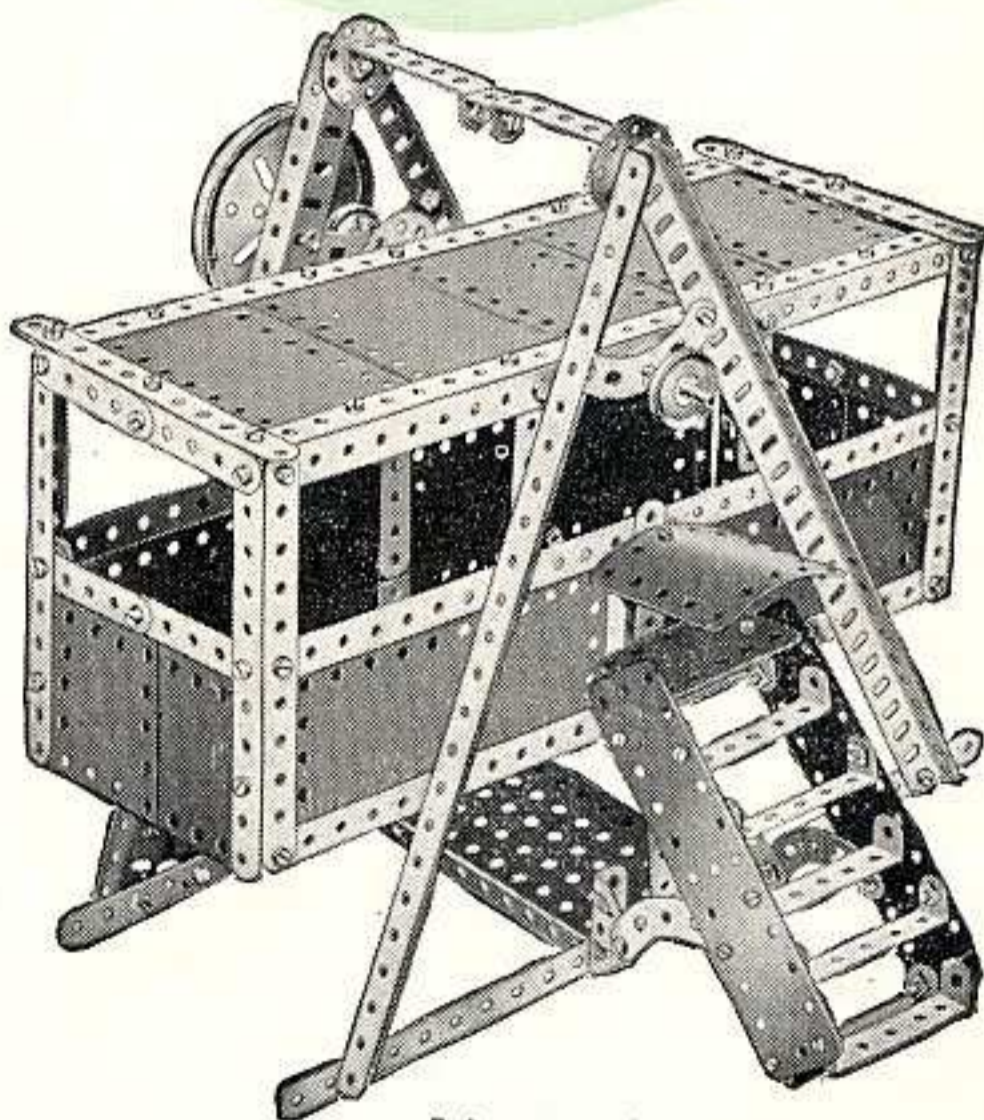
Balancoire géante Reusachtige schommelboot
