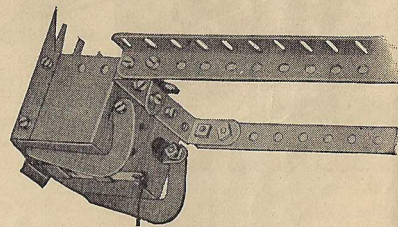
FIG. 4.61A. Comme l'indique cette gravure, on peut munir le bras du modèle d'une Pelle d'Excavateur Meccano (pièce No. 169.)
