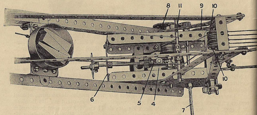
FIG. 4.45A. La machinerie vue de-dessus
