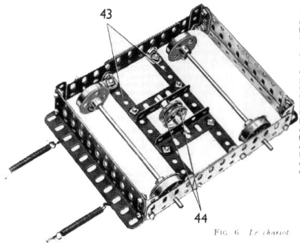
Fig. 6. Le chariot
