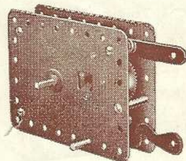
Moteur à ressort No. 1
